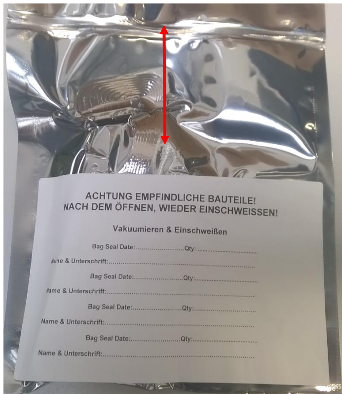
20) Einschweißte und etikettierte Rohleiterplatte
